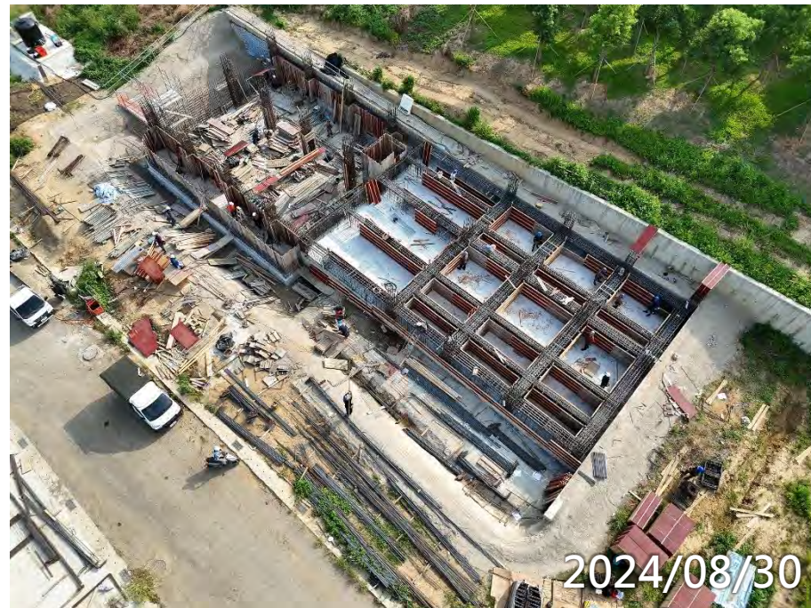
男義工低版區B1F、高版區地梁 鋼筋模板水電施作
