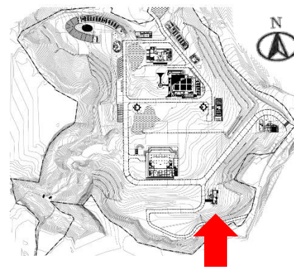
司機休息室土方開挖
