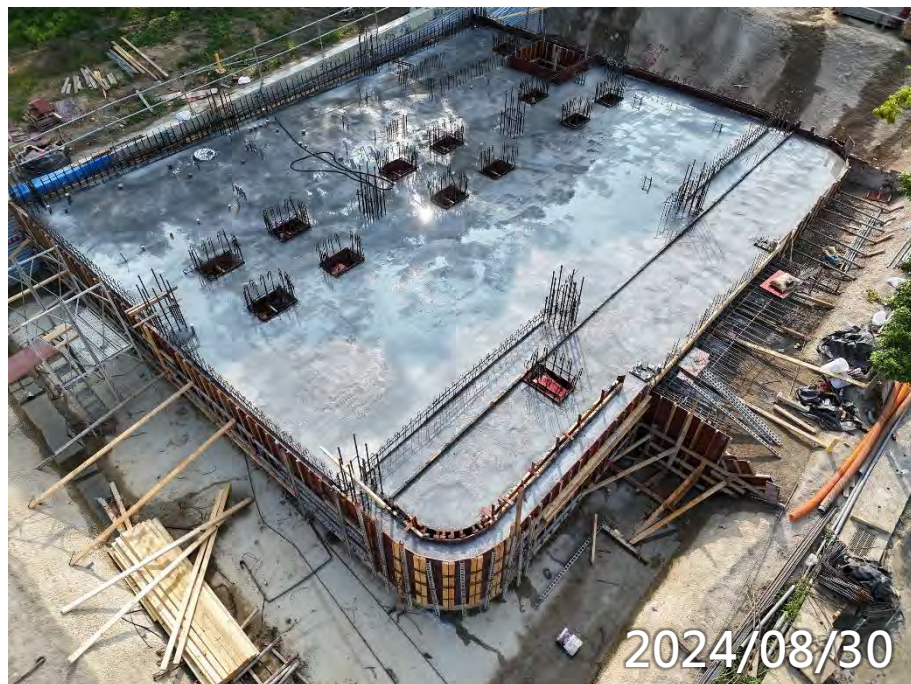
男常住BS版混凝土澆置
