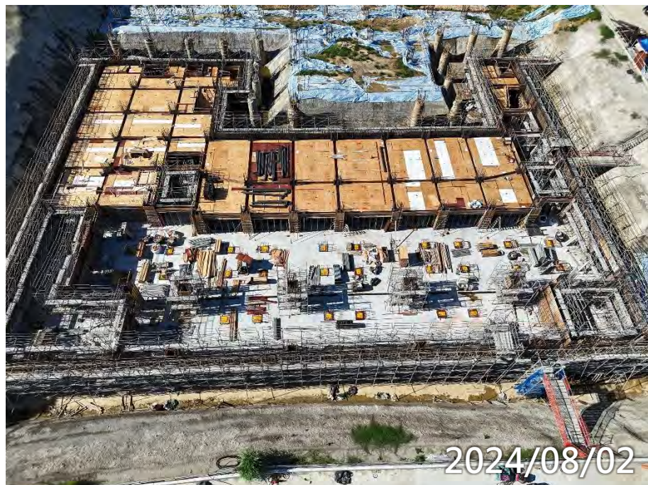
主殿1區B2F柱牆、B1F梁版 鋼筋模板水電施作
